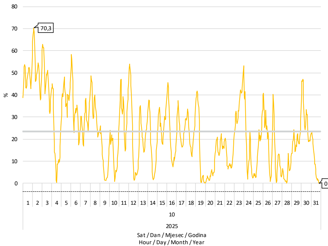
Slika 8 Udio proizvodnje vjetroelektrana u pokrivanju satnog opterećenja elektroenergetskog sustava u listopadu 2025. godine
