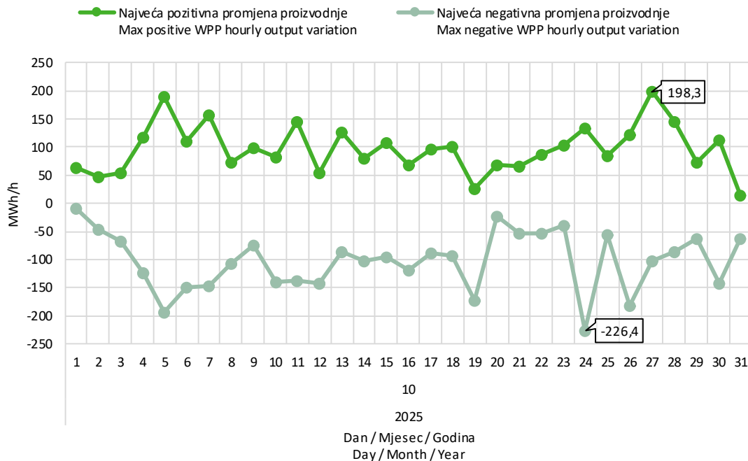
Slika 9 Maksimalna pozitivna i maksimalna negativna promjena satne proizvodnje VE u listopadu 2025. godine
