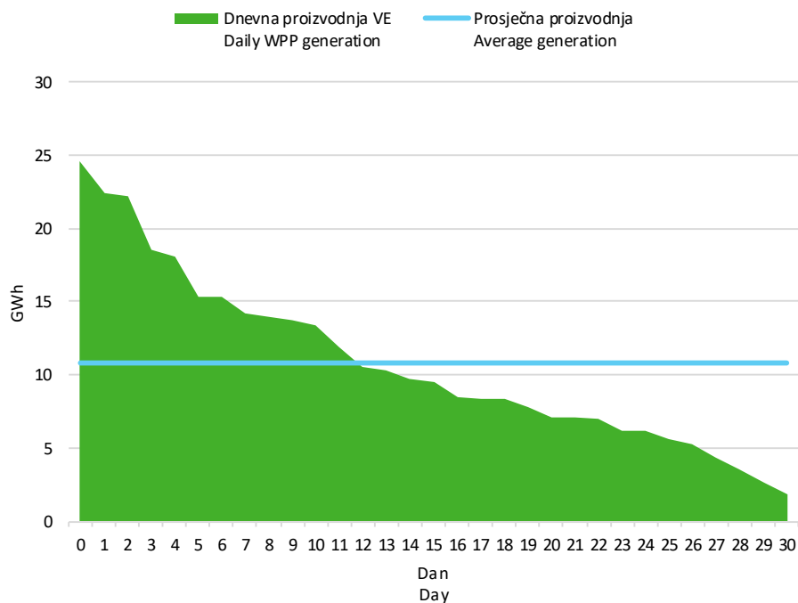
Slika 6 Krivulja trajanja dnevne proizvodnje vjetroelektrana u listopadu 2025. godine
