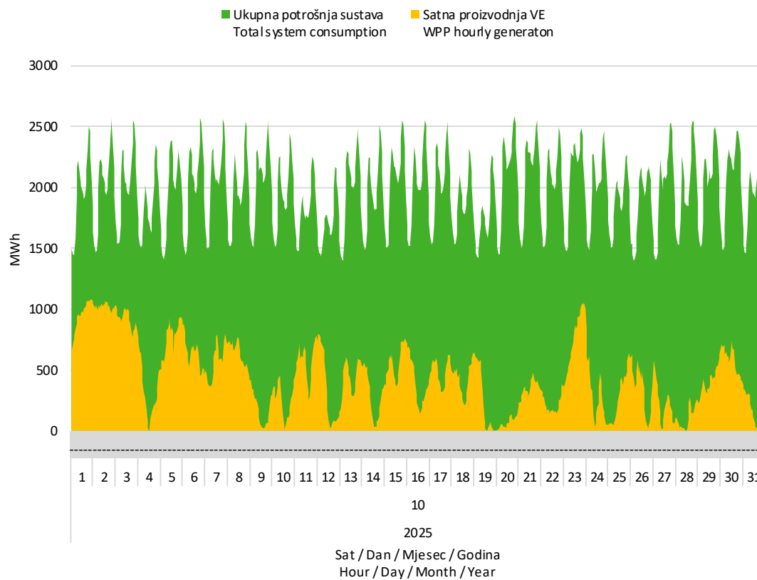
Slika 7 Usporedba satnog dijagrama opterećenja sustava i proizvodnje vjetroelektrana u listopadu 2025. godine
