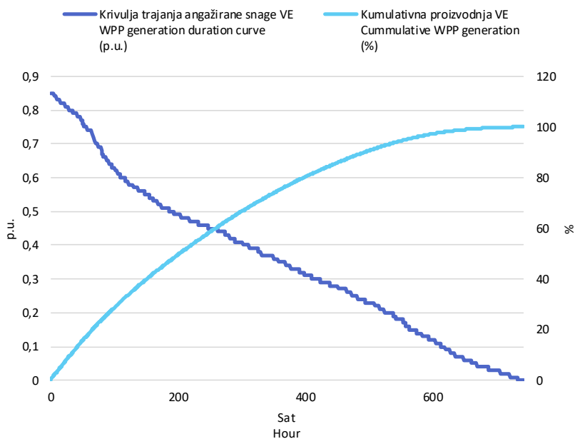
Slika 3 Krivulja trajanja angažirane snage svih VE i kumulativna proizvodnja VE u listopadu 2025. godine u jediničnim vrijednostima
