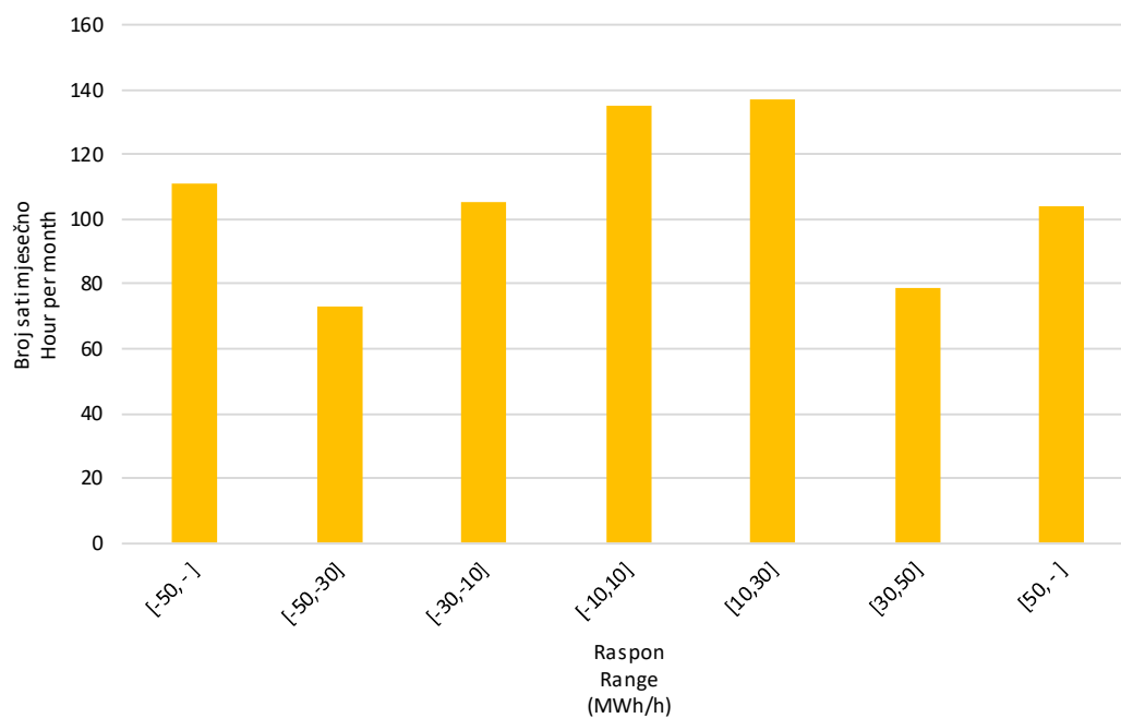
Slika 10 Statistička raspodjela satnih promjena proizvodnje VE u listopadu 2025. godine
