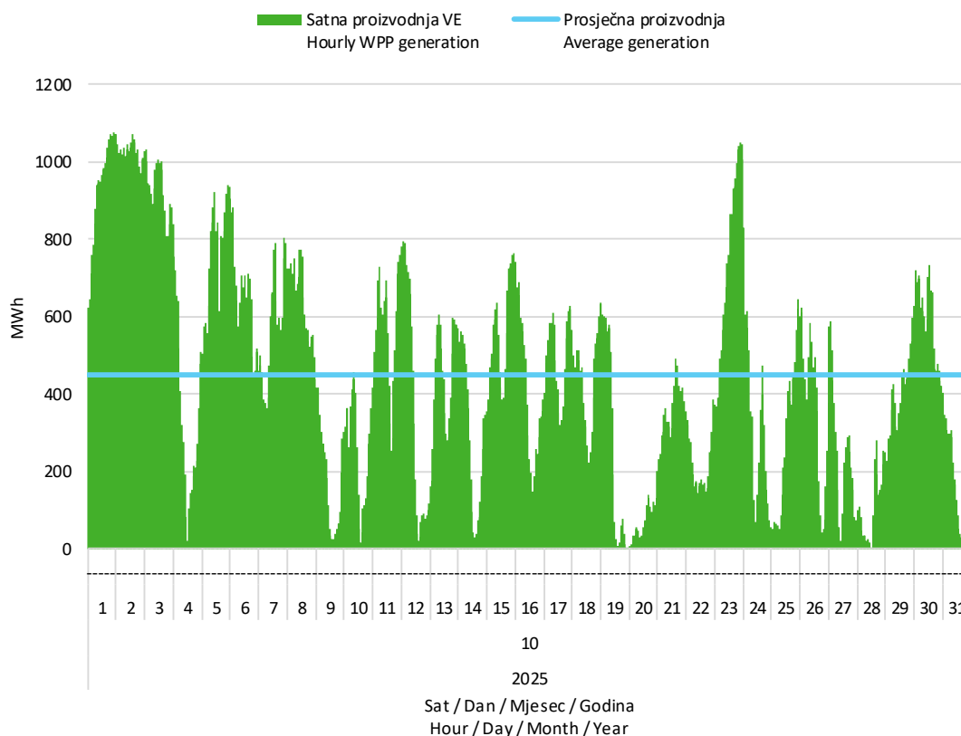
Slika 2 Satna proizvodnja svih vjetroelektrana u listopadu 2025. godine
